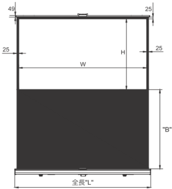
前面図
