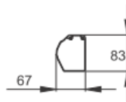
ケース側面図
